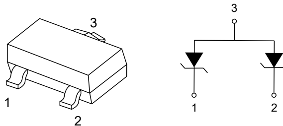
SOT-23
