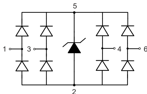
SOT-363
