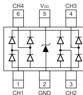
SOT23-6
