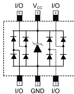
SOT-363
