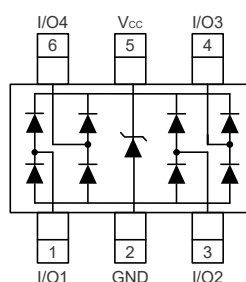
SOT23-6
