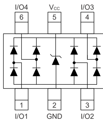
SOT23-6
